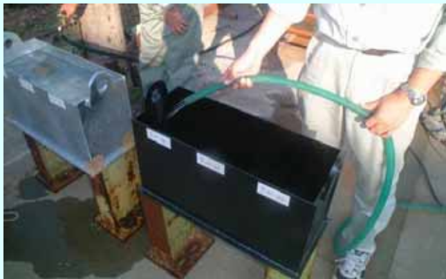
水張り試験状況
