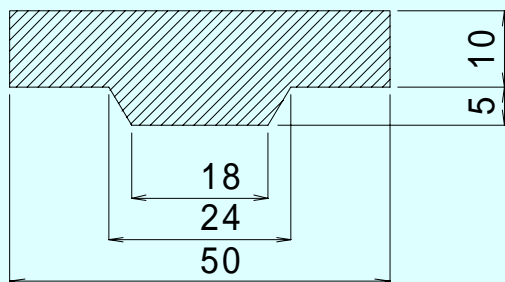
図．しょうかせんの基本寸法（実寸）
